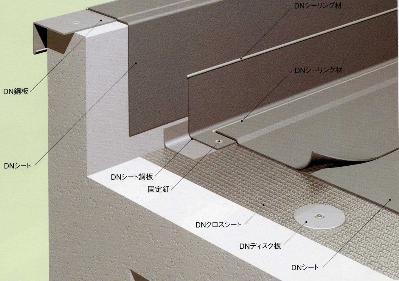
露出工法
